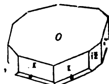
Binnenthal.
